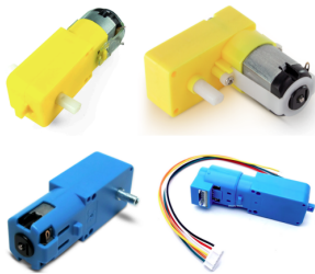
Figura 6. Motor tipo 130 com caixa de redução.
