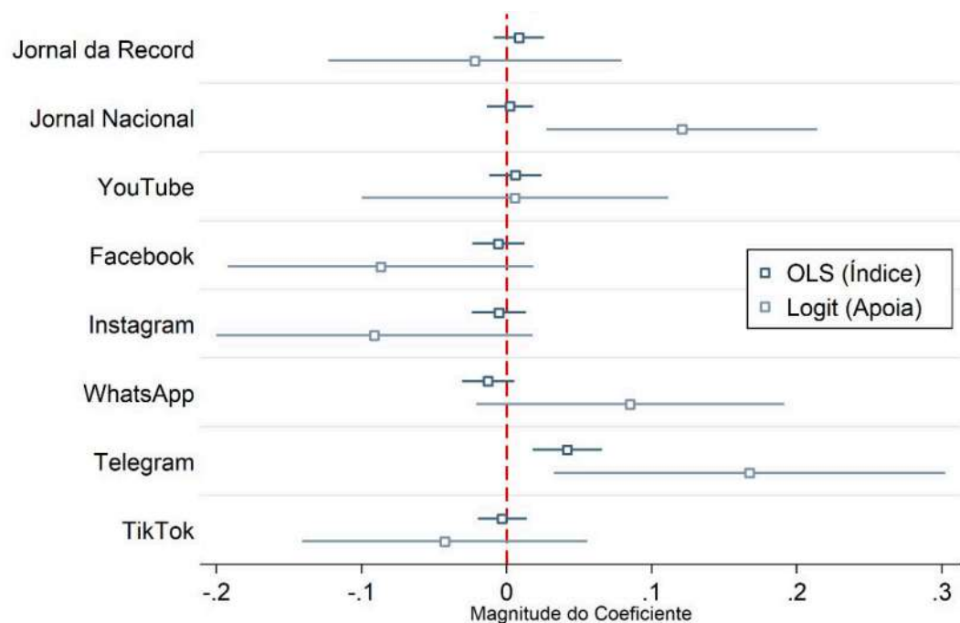
Figura 9 - Preditores de apoio à violência (mídia)
