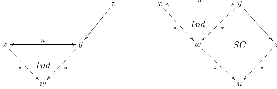
Figura 4.4.1: Semi-confluência implica a propriedade Church-Rosser
