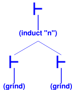
Figura B.1: Árvore de prova do teorema closed_form
