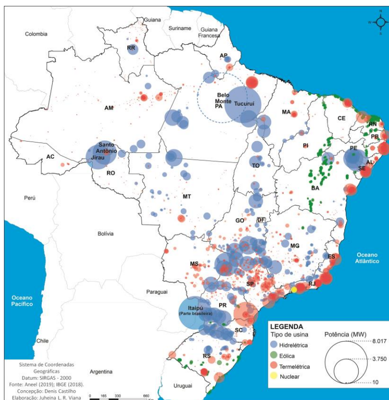
Figura 1. Distribuição das usinas geradoras de eletricidade no Brasil (2019)
