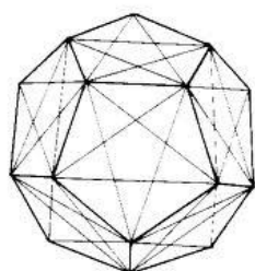
Figura 9 – Dodecaedro. Fonte: Mundo da leitura 52
