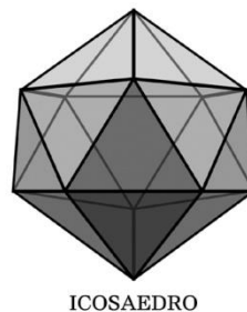
ICOSAEDRO Figura 10 – Icosaedro. Fonte: Aulete digital 53
