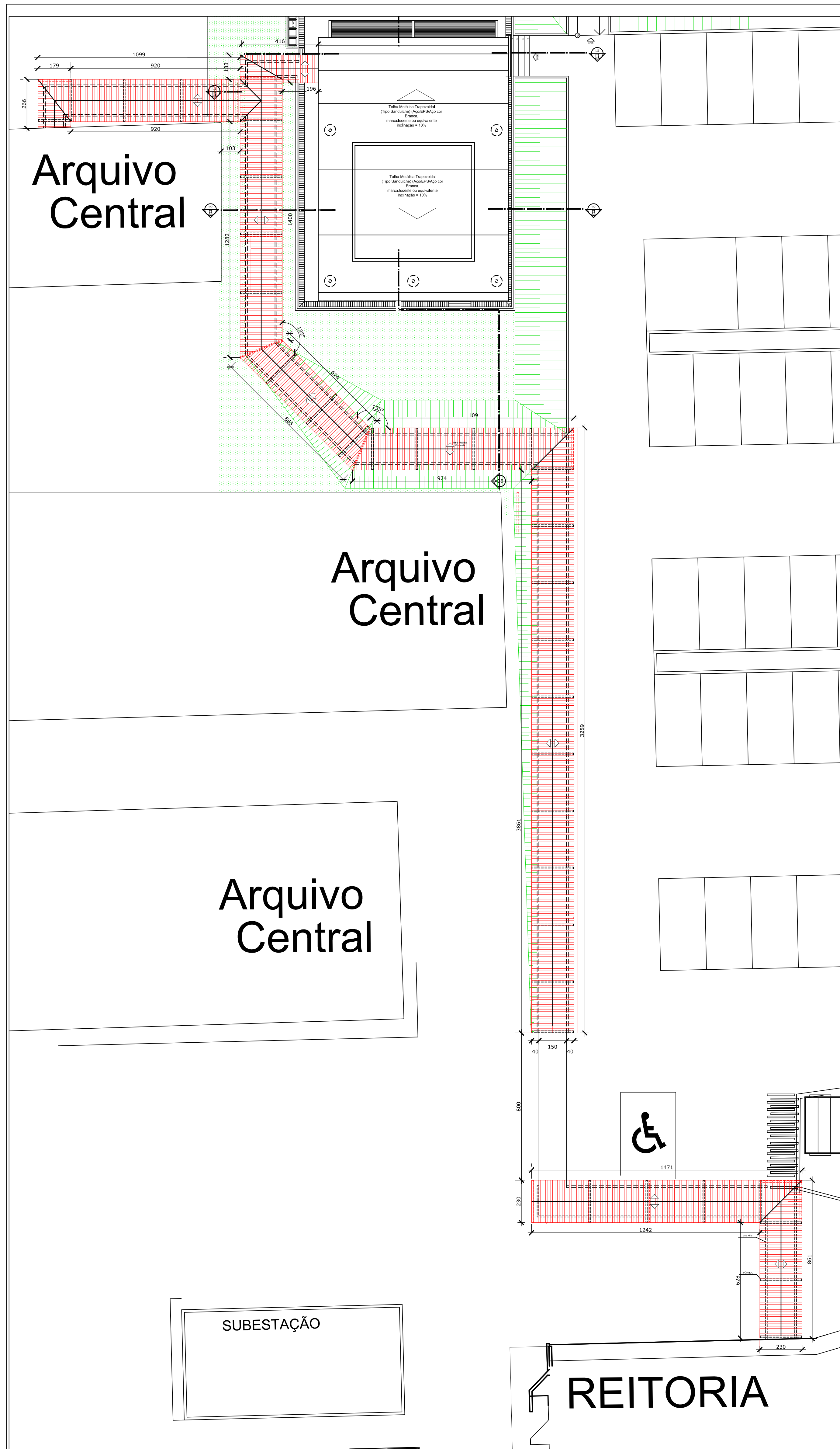
PLANTA COBERTURA PASSARELA ESC.1:125
