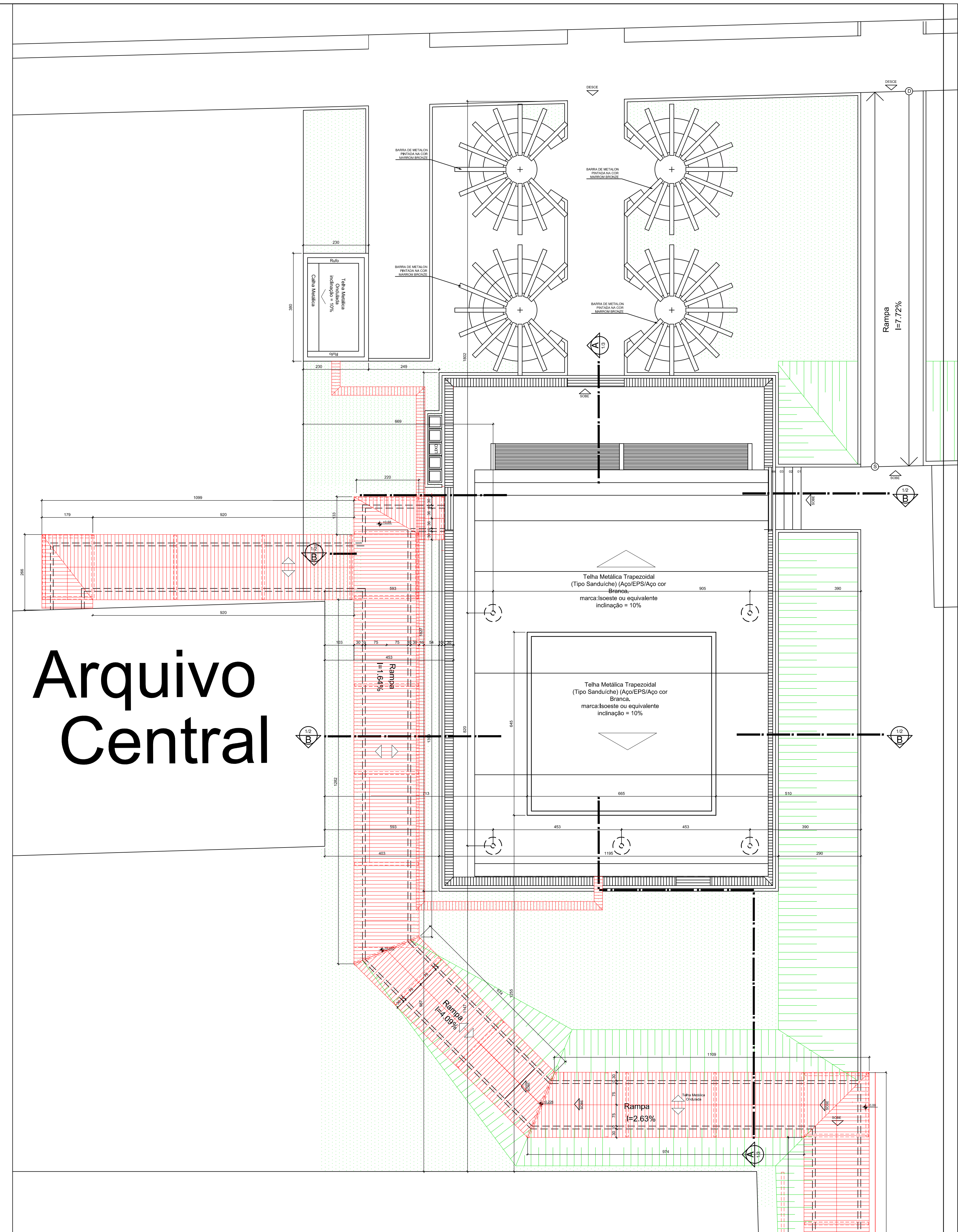
PLANTA DE COBERTURA ESC.1:75
