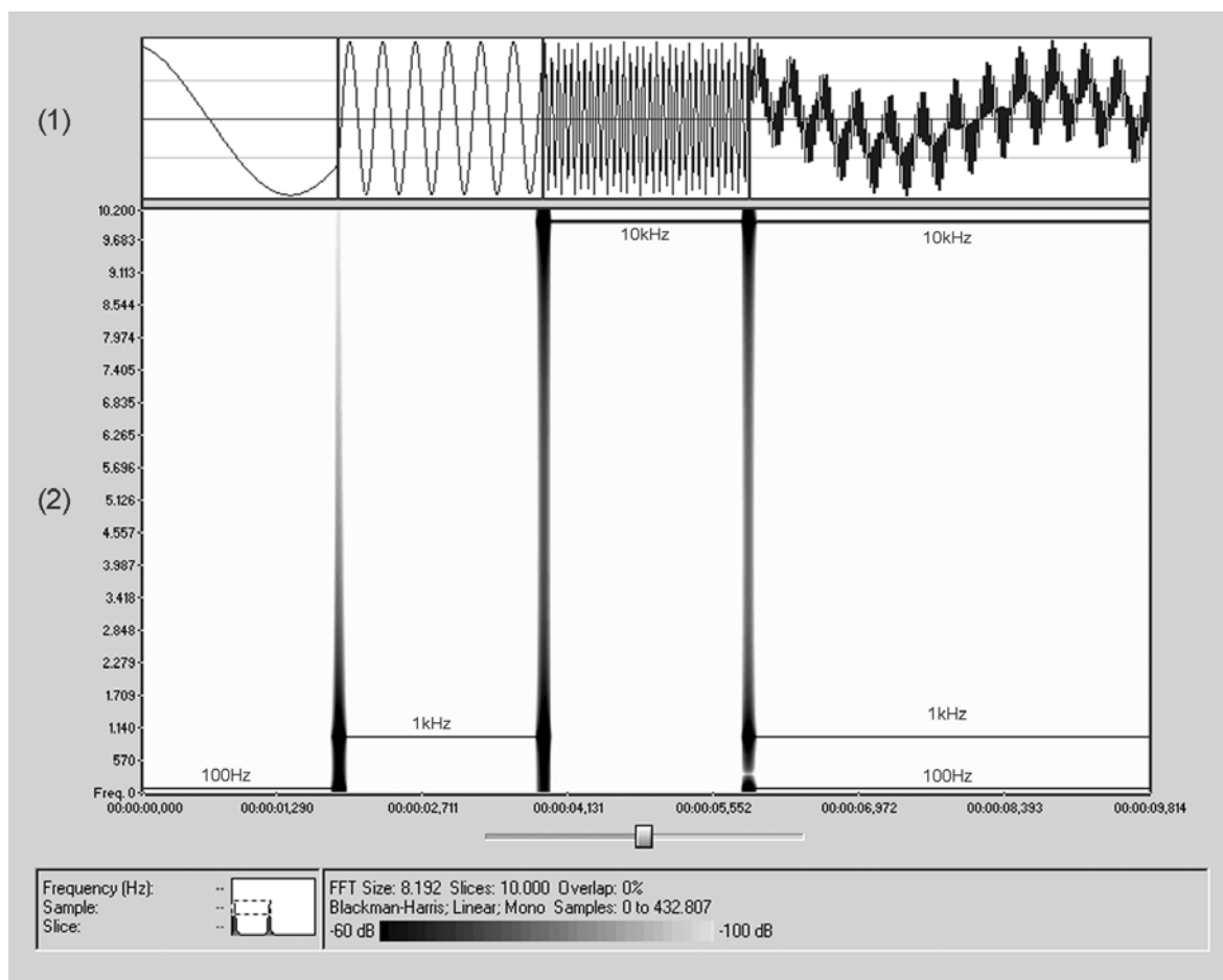
Imagem 2 – Sonograma e espectrograma de três oscilações harmônicas simples e da oscilação complexa composta por elas. Temos acima: (1) uma seqüência sonográfica de trechos de três tons puros de 100Hz, 1kHz e 10kHz e de um tom composto pelas mesmas três freqüências; e (2) um espectrograma correspondendo a trechos proporcionais da mesma seqüência de freqüências do sonograma (cf. Exemplo Sonoro 30 ). O espectrograma é um gráfico tridimensional no qual o eixo vertical exibe as freqüências encontradas no som, o horizontal exibe a sua duração temporal e o de profundidade exibe a sua intensidade (representada pelos tons de cinza, que vão do fundo branco menos intenso à superfície preta mais intensa). Seria como girar perpendicularmente com relação ao sonograma e passar a vê-lo de cima (ou de baixo) – pois aquilo que no sonograma é o eixo vertical (intensidade) se torna, no espectrograma, o eixo da profundidade –, como passar a ver uma cadeia de montanhas de cima e não do nível do chão – de forma que as vibrações que eram sobrepostas umas às outras no sonograma se espalham em linhas distintas no espectrograma. O espectrograma poderia ser descrito como um sonograma acrescido de uma dimensão, a das freqüências, e sua vantagem com relação ao sonograma é não apenas a possibilidade de obter uma representação visual da variação de freqüências mas, principalmente, de obter essa representação de maneira precisa (pois no sonograma vemos apenas a diferença nos comprimentos de onda, mas não o valor das freqüências representadas). O espectrograma é produzido através de uma série de decomposições analíticas (conhecidas como análise de Fourier) de curtos trechos de um som complexo em suas freqüências simples constituintes (cf. Lehiste 1987:282; Courtney 1992; Engelson 1999; Charley et al. 2001; Schafer 2001:178-9). As três faixas verticais que aparecem nas
